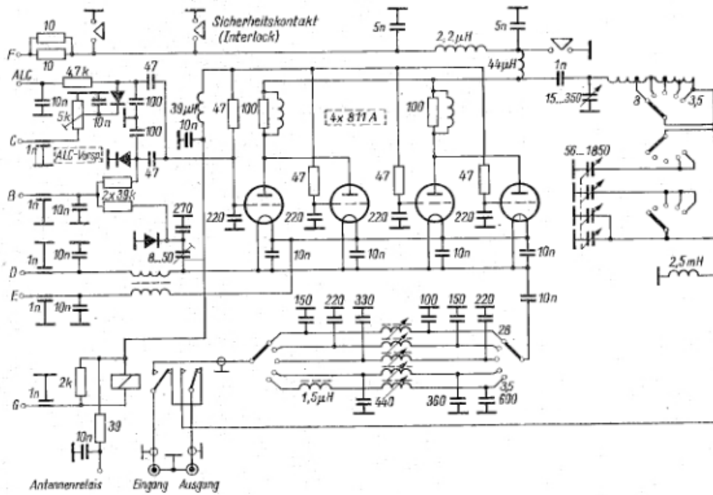
•Bild 16.70 (a und b) Linearverstärker Collins 30 L-1
