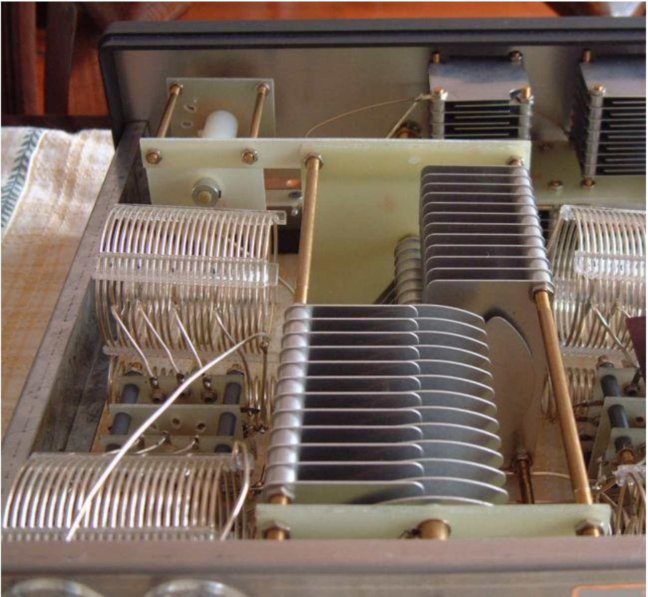
Bovenzijde vanaf achterkant
