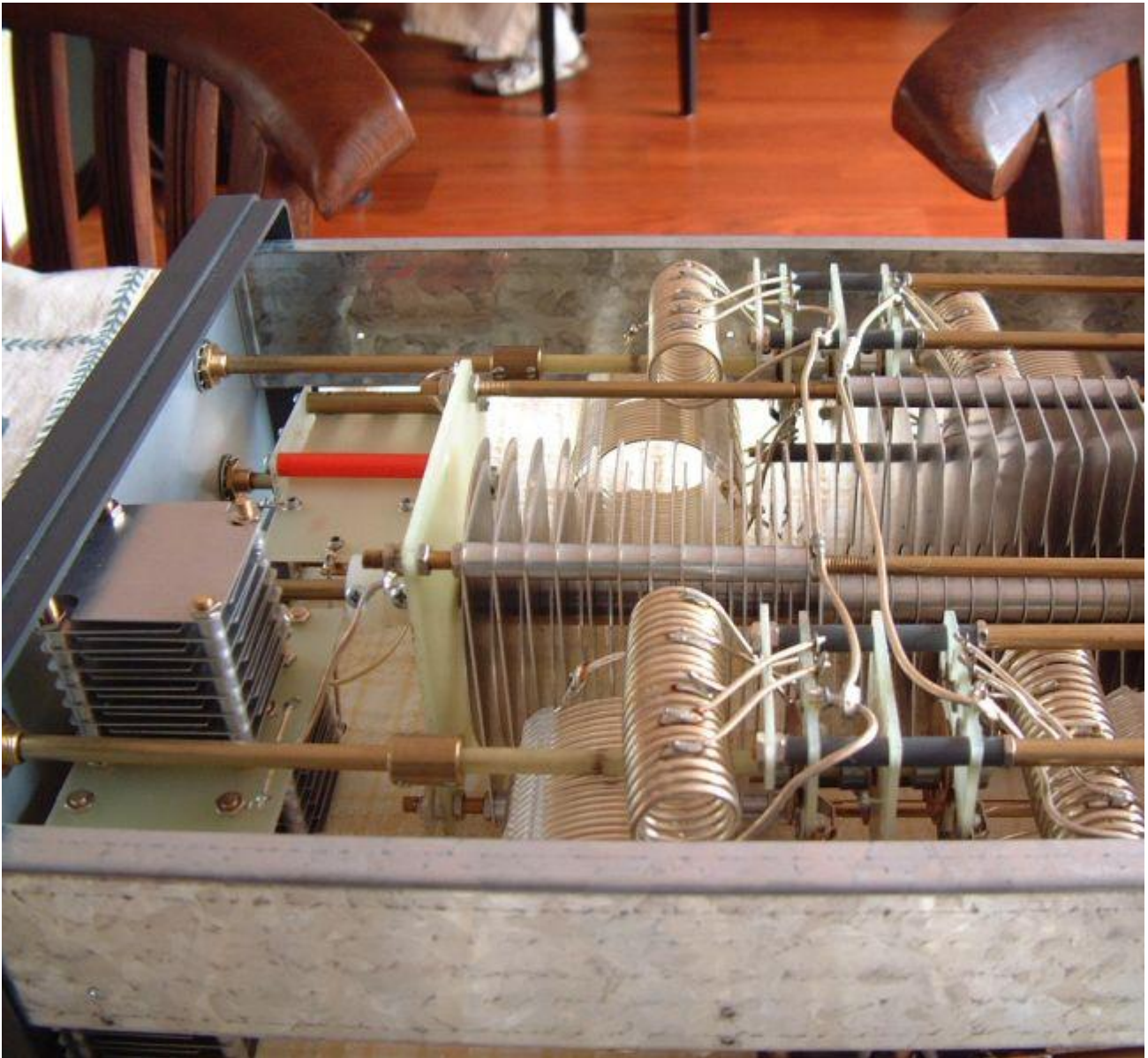
Onderzijde vanaf zijkant links
