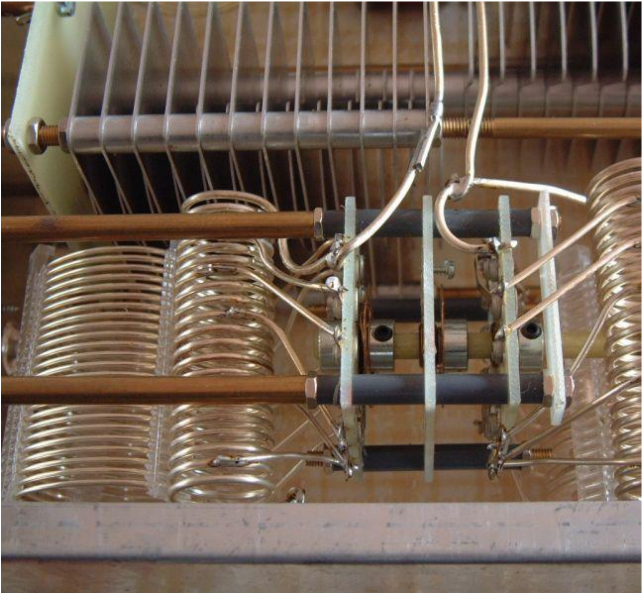
Schakelaar 1 vanaf onderzijde
