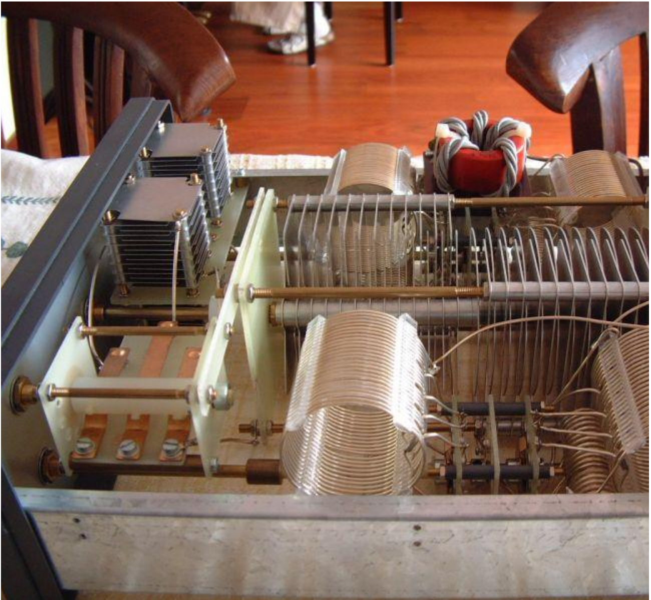
Bovenzijde vanaf zijkant rechts
