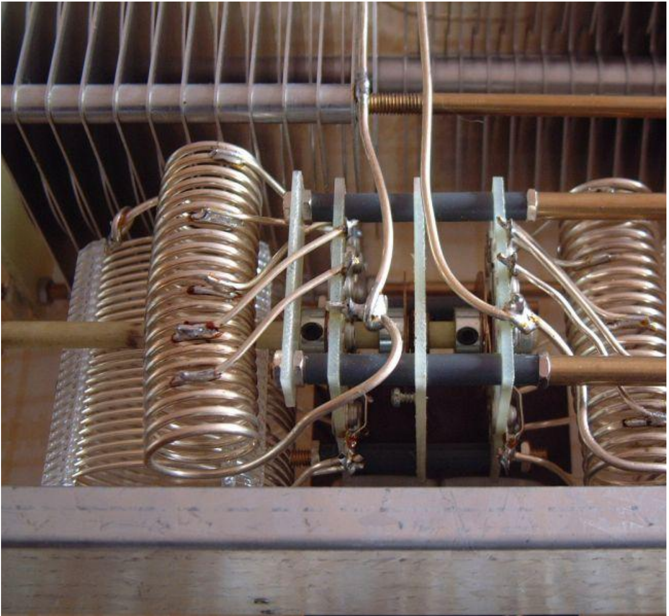
Schakelaar 2 vanaf onderzijde
