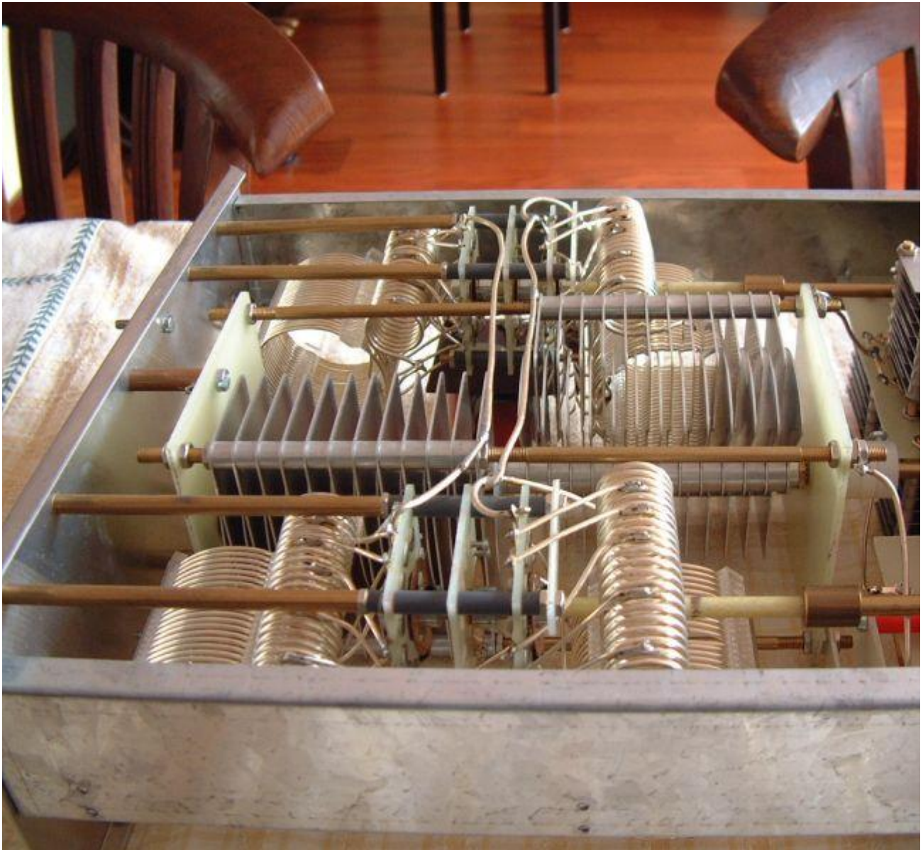
Onderzijde vanaf zijkant rechts
