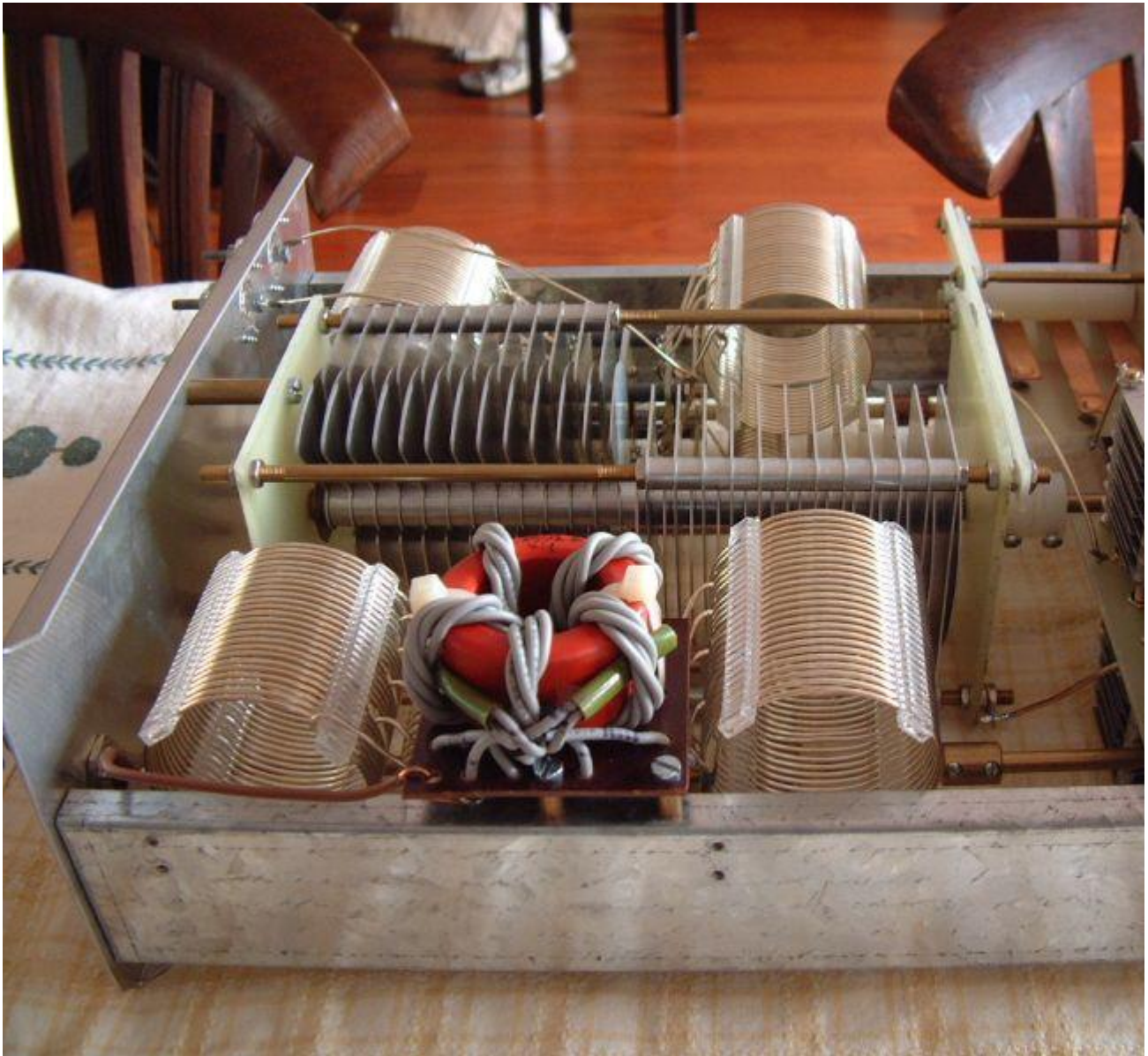
Bovenzijde vanaf zijkant links
