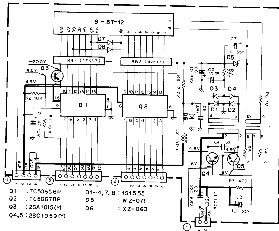
DISPLAY (X54-1630-00)
