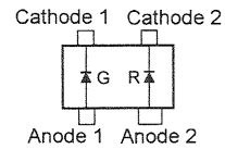
SML-020MLTT86 (D9918)
